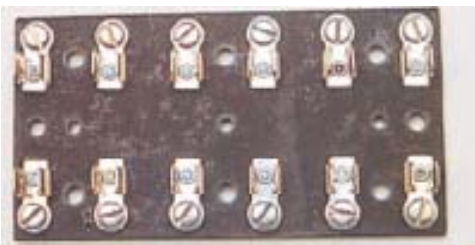
766023 6 FUSIBLES
